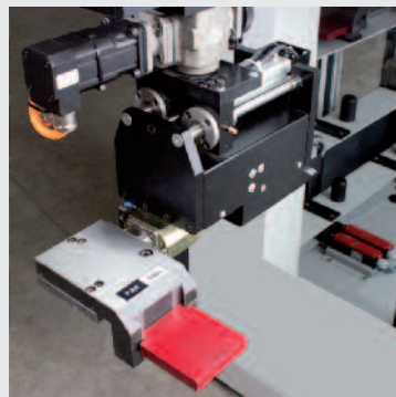
Nullpunktgreifer beim Drahterodieren
