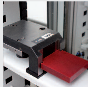
Herstellerunabhängiges Palettenhandling
